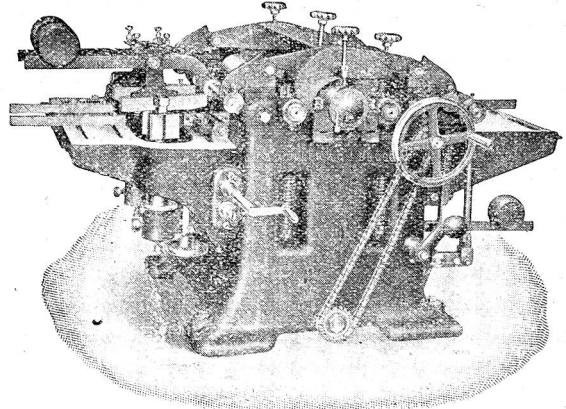
Dreseitige Hobelmaschine.
