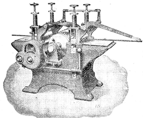
Latten-Kreissäge
