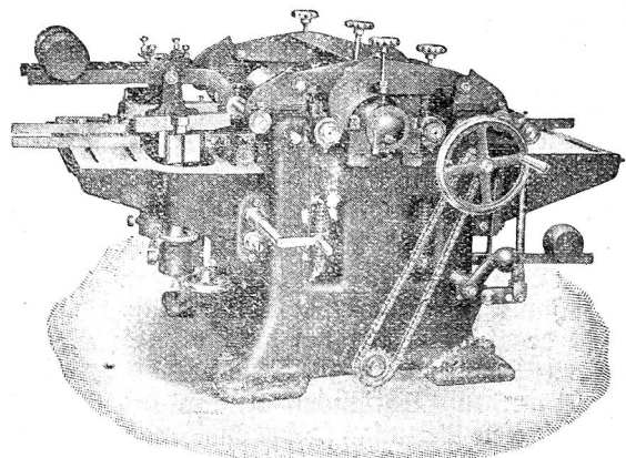
Dreiseitige Hobelmaschine.
