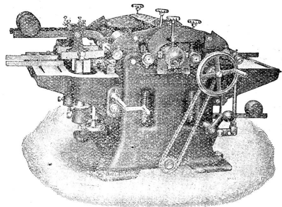
Dreiseitige Hobelmaschine.
