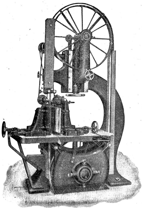
Trenn-Bandsäge mit selbsttätigem Walzeneinzug.
