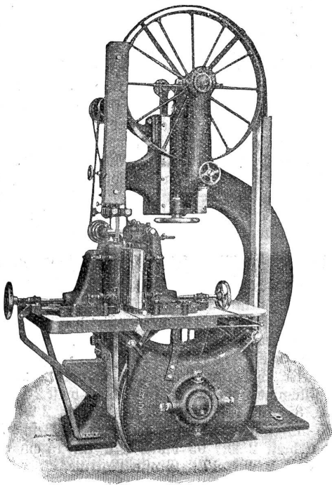
Trenn-Bandsäge mit selbsttätigem Walzeneinzug.
