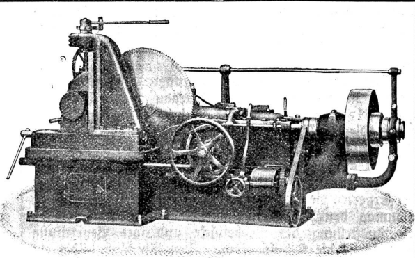
Schnell-Kaltsägemaschine SS.
