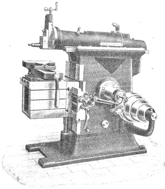
Shapingmaschine 450 mm Hub sowie alle andern Werkzeugmaschinen
