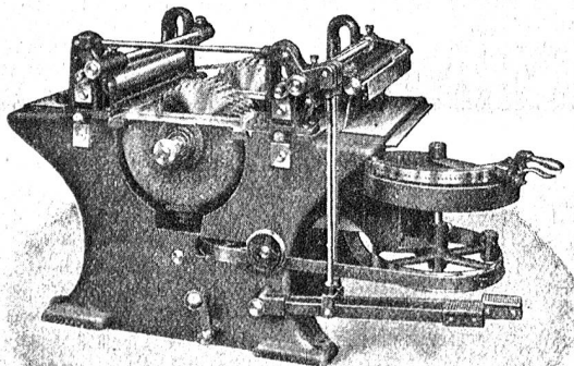
Doppelte Besäum- und Lattenkreissäge mit selbsttätigem Vorschub
