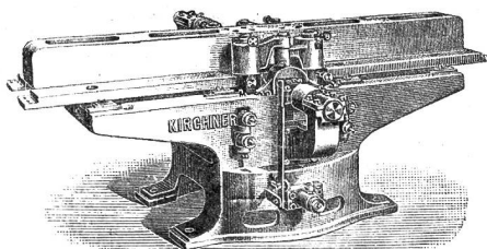
Nut-, Spund- und Fügemaschine für konische und parallele Bretter
