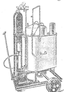
Grobstück-Apparat „Nova“
