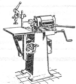
Riemenlose Langlochbohrmaschine
