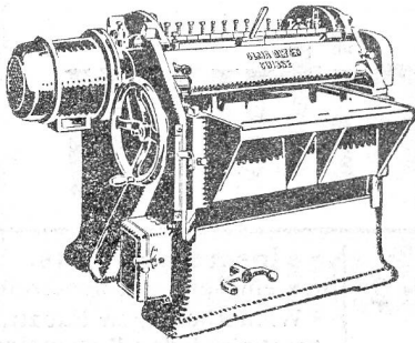
Riemenlose Gliederwalzen-Dickenhobelmaschine.
