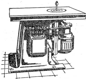
Riemenlose Kehlmaschine
