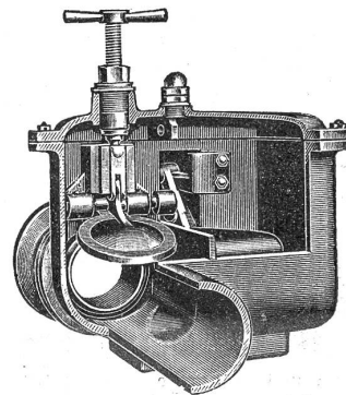
RÜCKSTAU-ABSCHLUSS
