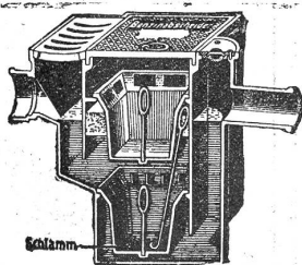
BENZIN-ABSCHIEDER
