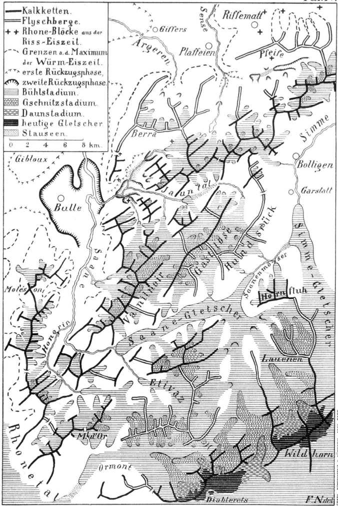
Gletscherkarte vom Saanegebiet.
