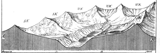
Fig. 3. Taltrog mit Talschluss im Flyschgebirge. Profil A-B ist gleich dem Querschnitt Blattenhorn - Arniensee - Arnihorn. Höhe Längsprofil UK - Ursprungskare SK - Seitenkare. Motive aus d. Tornellan-Gruppe.
