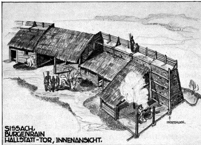
Hallstatt D. Burgenrain. Wehrmauer mit Wehrgraben und Brustwehr, rechts im Schnitt. Hütten auf der Innenseite, links der Mitte die Toranlage. — Trockenmauer- werk, mit Pfosten und Balken armiert (murus gallicus nach Cäsar). Von Ad. Müller gezeichnet nach Angaben von Dr. E. Vogt.
