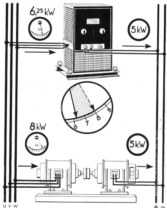
Schematische Darstellung der Wirtschaftlichkeit eines Kino-gleichrichters gegenüber der Umformergruppe.
