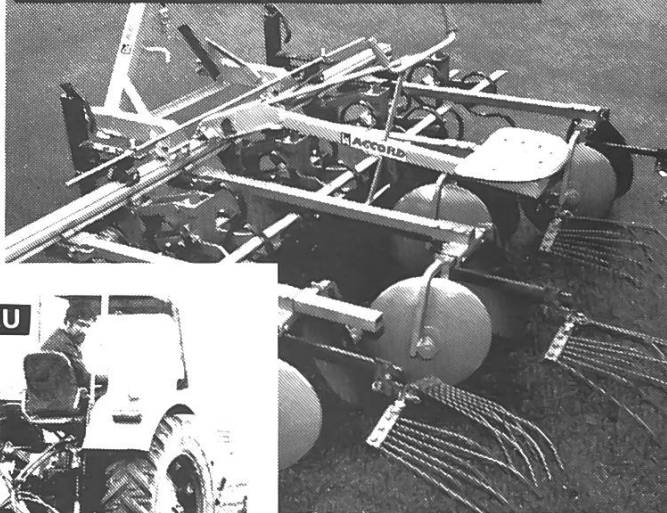
Hack- und Häufelgeräte 2- und 4reihig
