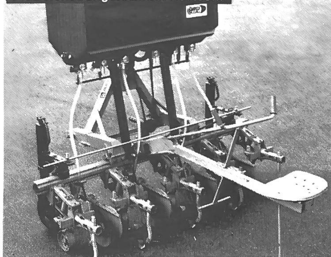
Präzisionsdüngerstreuer Bärtschi
