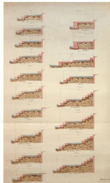
Plan Nr. 4 Querprofile, A.H. Hünerwadel (1856)
