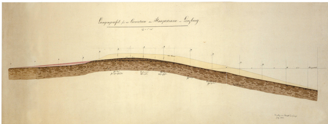
Plan Nr. 5 Längsprofil, Baumeister Wolf (1856)
