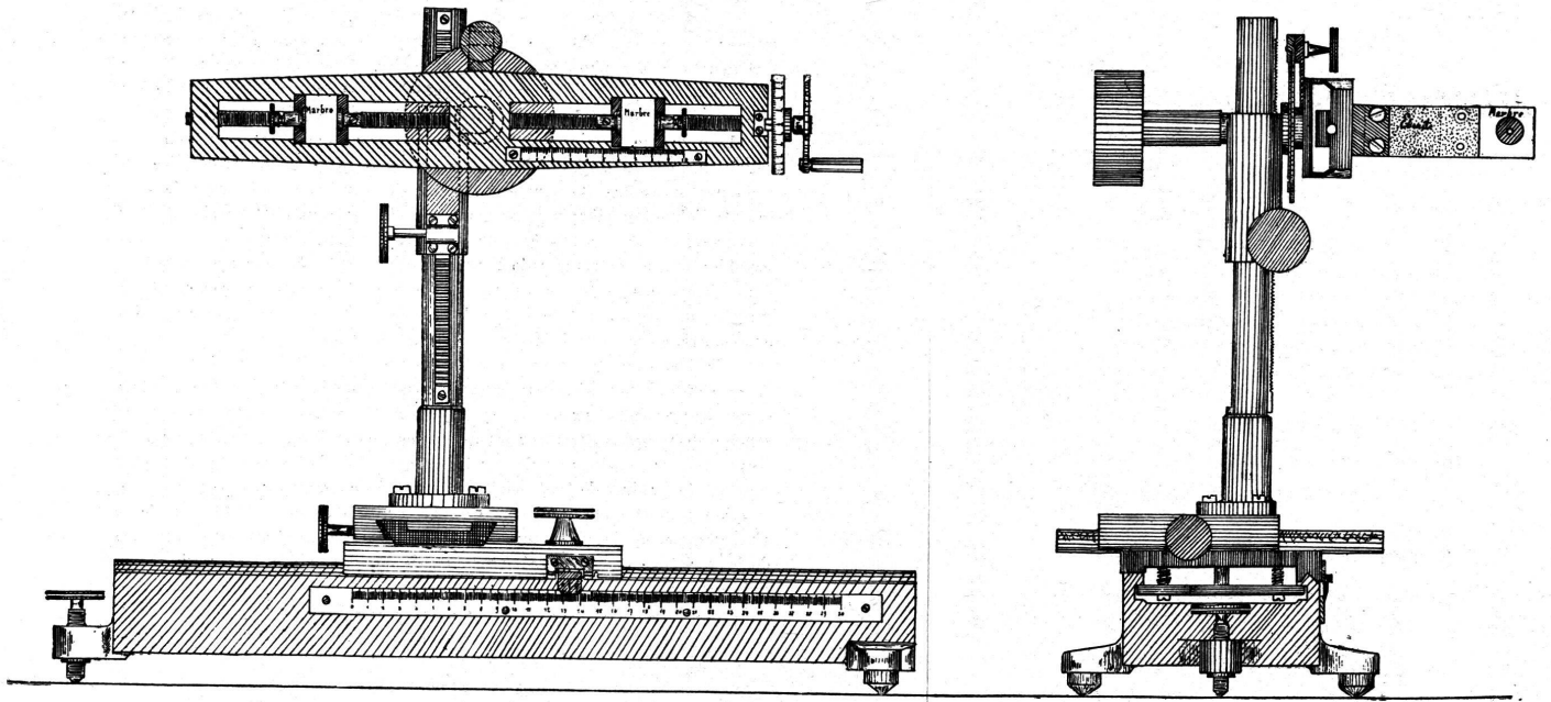
Figure 26: Spectro-déflagrateur de précision (échelle \frac{1}{4} )
