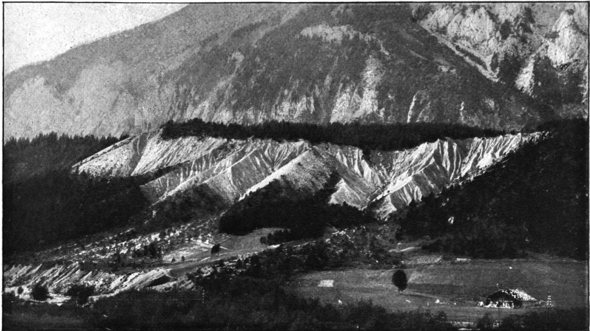
Fig. 4. Die erodierten Bergsturzmassen von auf „der Höh“ bei Kandersteg.
