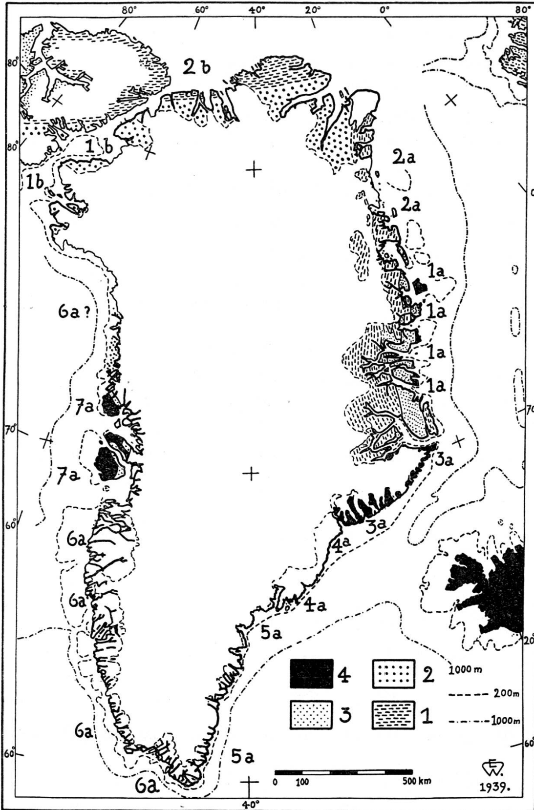
Abb. 1. Tektonische Skizze von Grönland.
