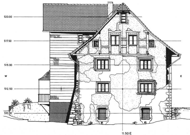
Aufnahmeplan der Südfassade.
