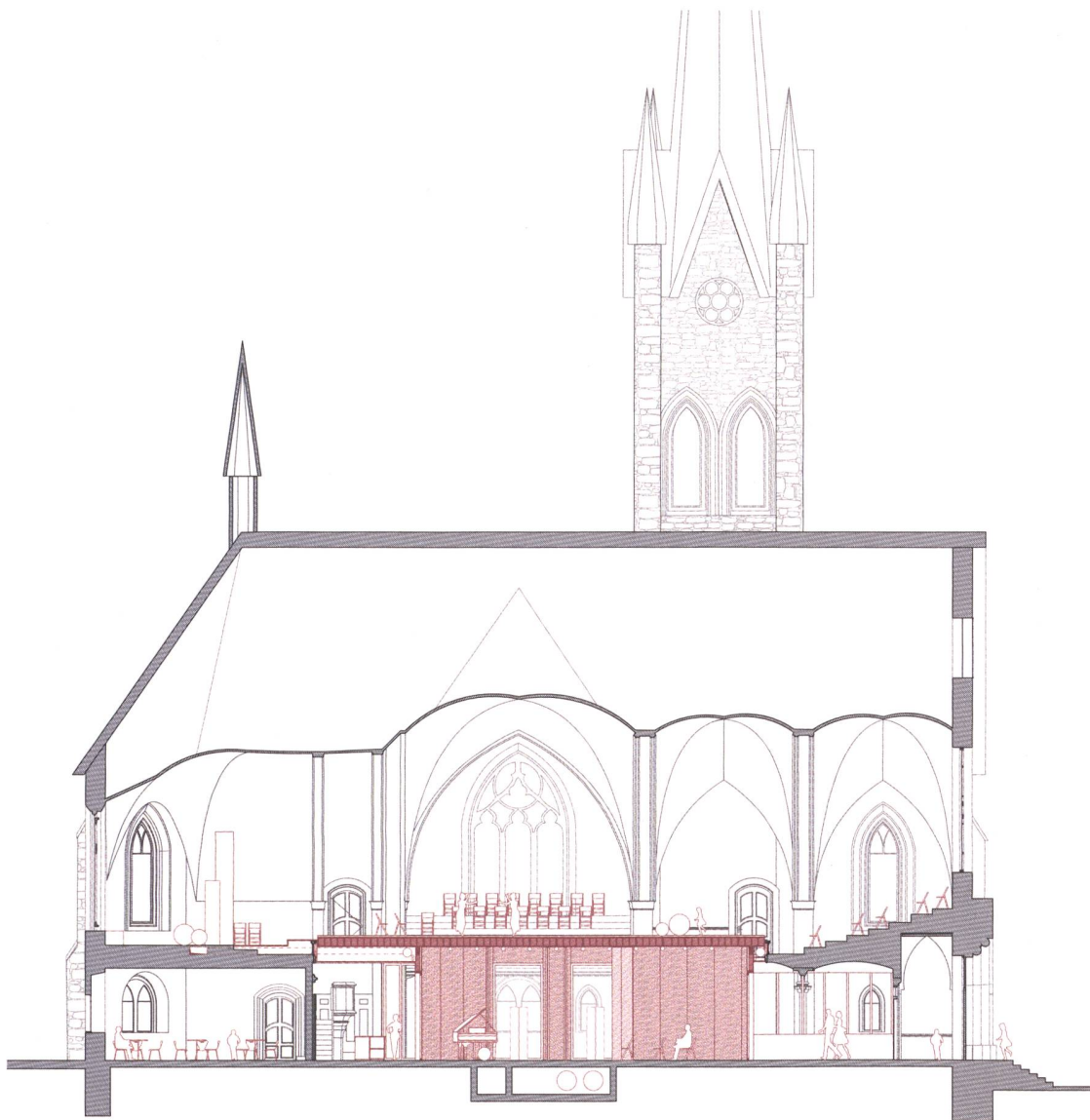
Längsschnitt. Die Umnutzung verändert den Kirchenraum, doch der Zeugniswert des Baudenkmal bleibt erhalten. © Vécsey*Schmidt Architekt*innen
