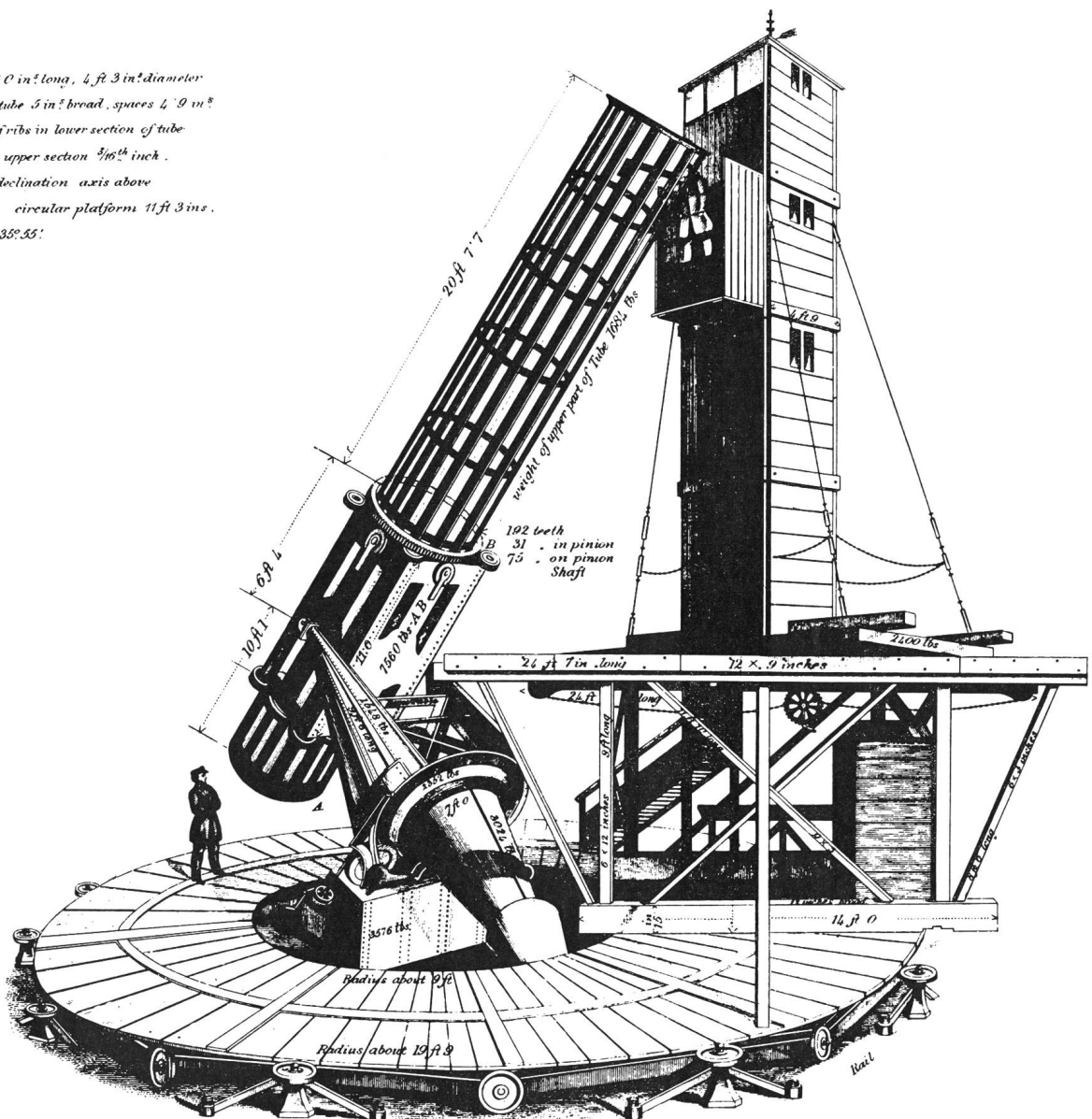
Abb. 2: Das grosse, von W. LASSELL selbst gebaute und um 1861–1864 in Malta aufgestellte Spiegelteleskop. Der ebenfalls von ihm selber geschliffene Spiegel hatte eine Öffnung von 120 cm und eine Brennweite von etwa 11 m 4 ).
