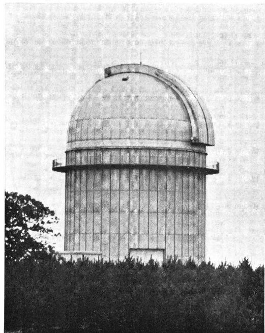
Abb. 2: Die Kuppel des 98-Zoll ISAAK NEWTON-Teleskops. Die Gesamthöhe dieses Gebäudes beträgt 28 m und die Kuppel allein wiegt 120 Tonnen.
