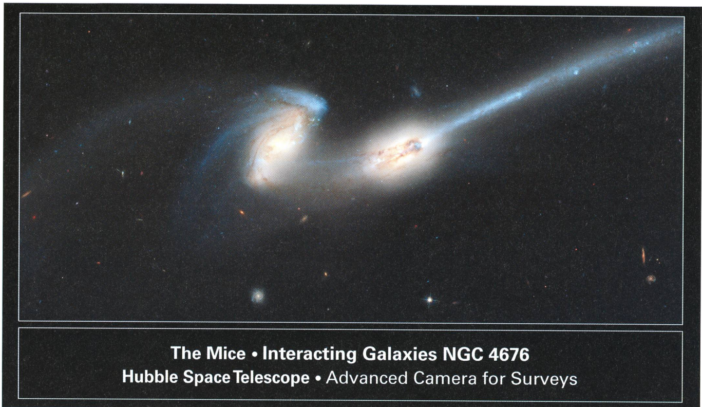
Bild 4: NGC 4676, Mäusegalaxien.
