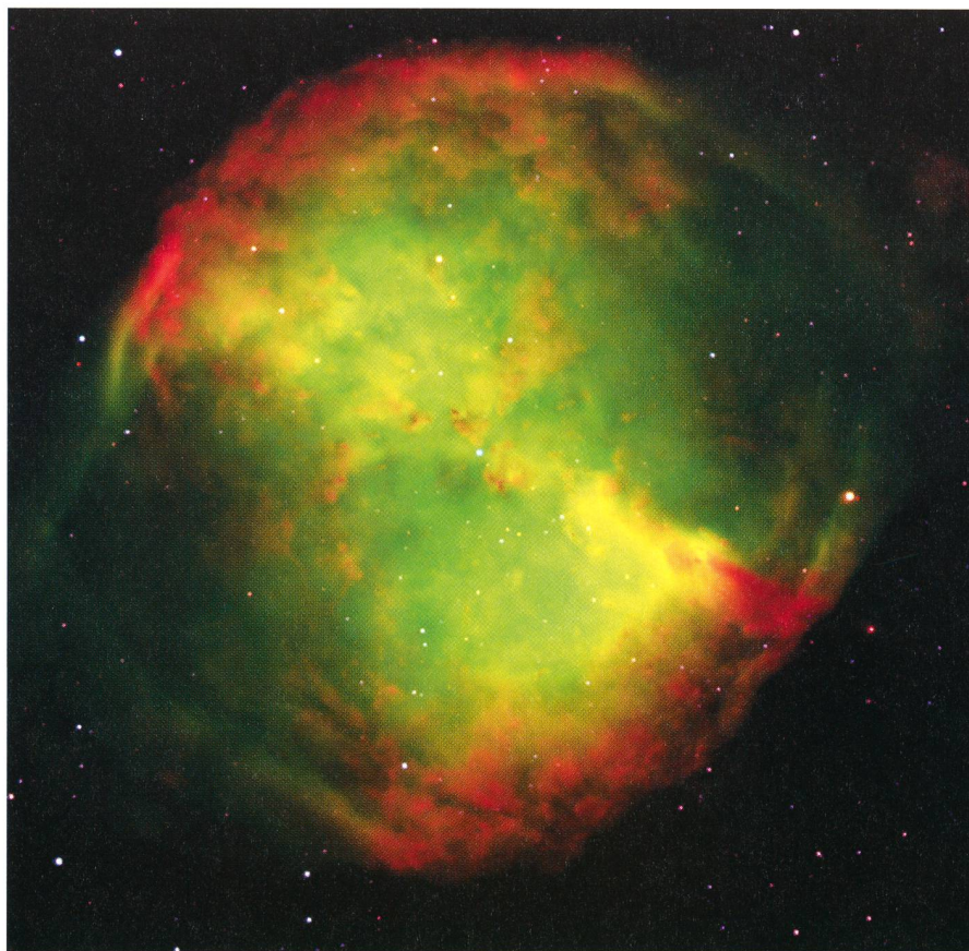
Fig. 13: La nébuleuse planétaire NGC 6853 (M27)(Photo VLT).
