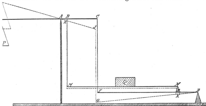
Brückenwage (Schematische)
