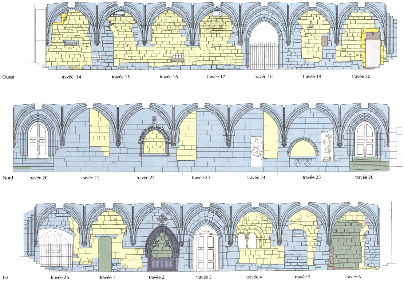
Fig. 133 Coupes longitudinales et élévations des murs des trois galeries du cloître. Abb. 133 Längsschnitte und Wandaufriss der drei Seiten des Kreuzgangs.
