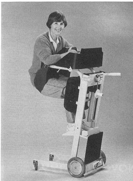
Unser Sitztransferlifter - der genialste Patientenheber.
