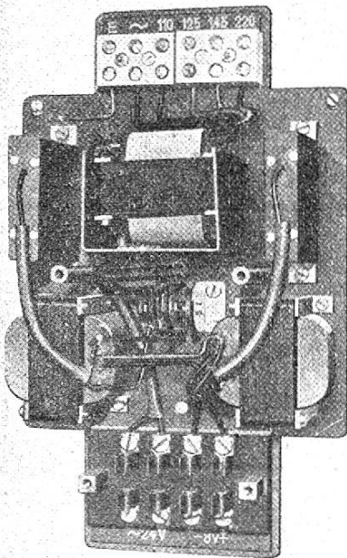
Speise-Gleichrichter
