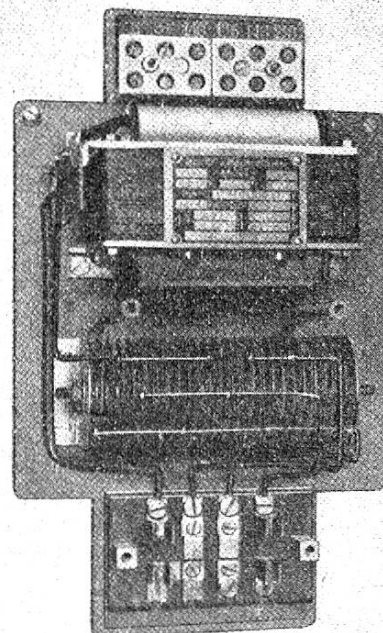
Signal-Gleichrichter
