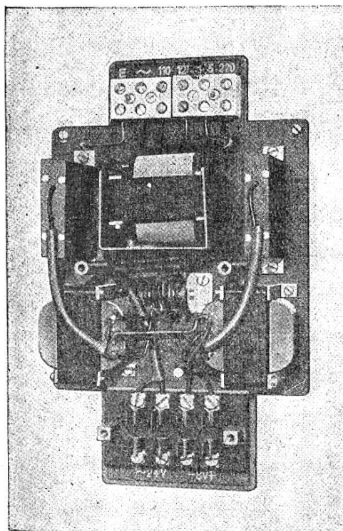
Speise-Gleichrichter
