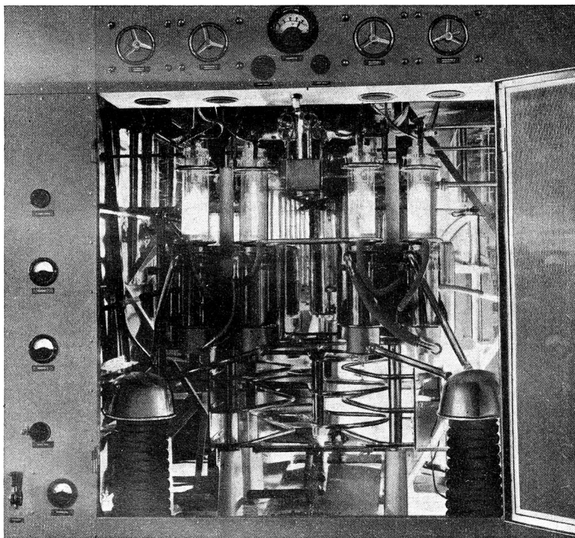
Kurzwellensender Schwarzenburg. Teilansicht einer 25—40-kW-Endstufe
