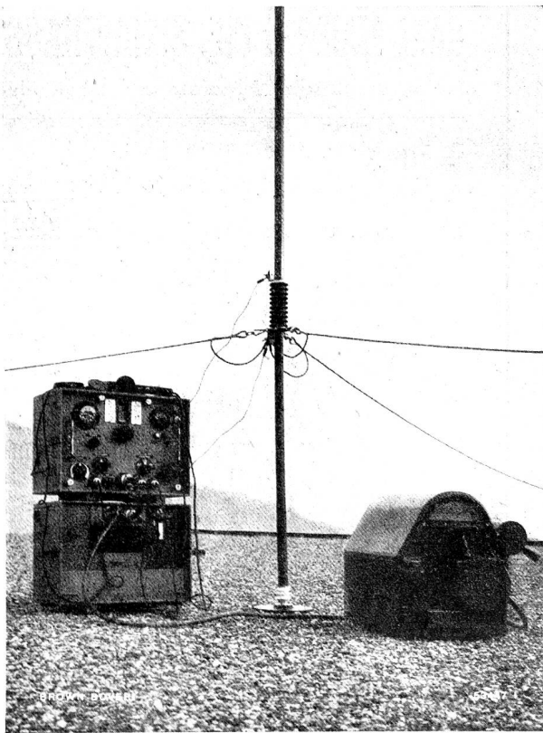
Tragbare leichte Sende-Empfangsstation mit benzinelekt. Aggregat
