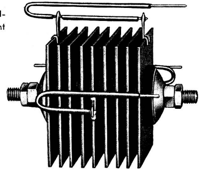
Kupferoxydul- Gleichrichterelement
