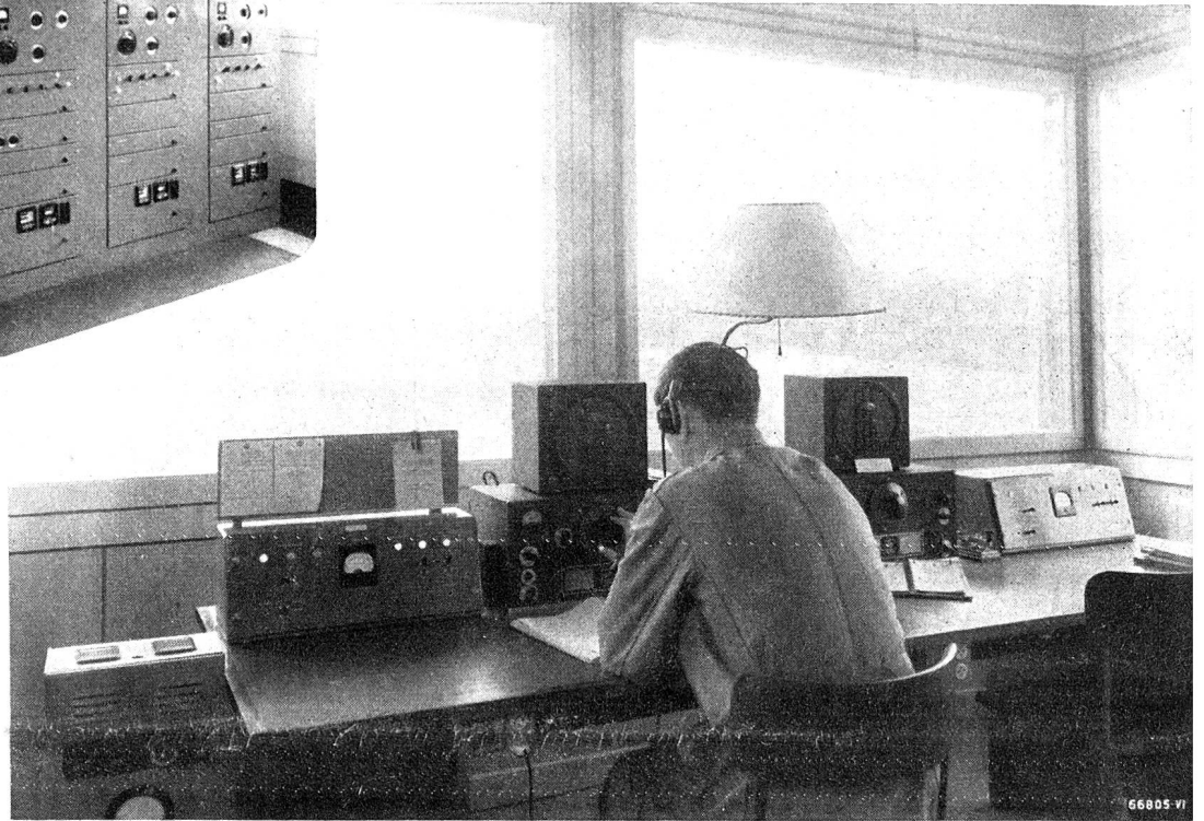
Vier zu einem Block vereinigte 300-W-Kurzwellensender in der Funkstation Avanche d. Flugplatzes Genf-Cointrin
