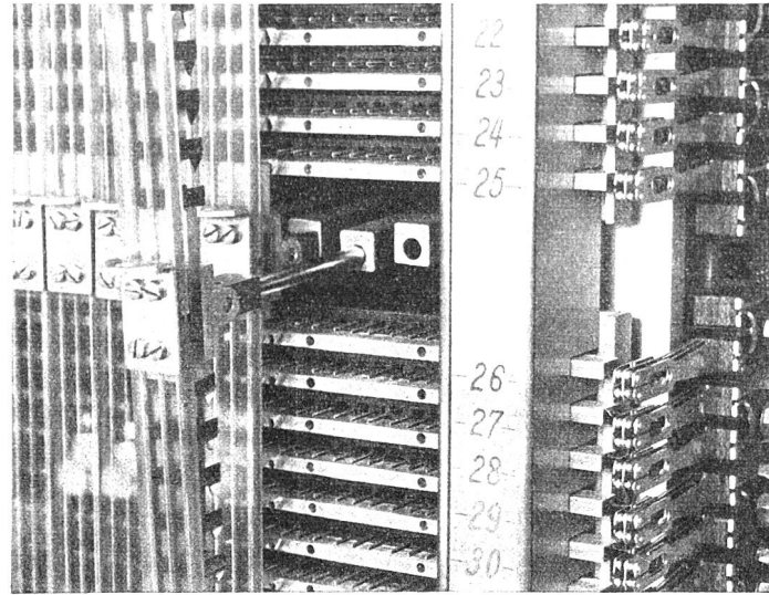
Ausschnitt aus dem Kreuzwähler mit ausgezogener Schaltstange
