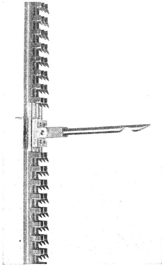
Schaltstange, Teilansicht
