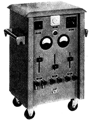
Fahrbarer Gleichrichter
