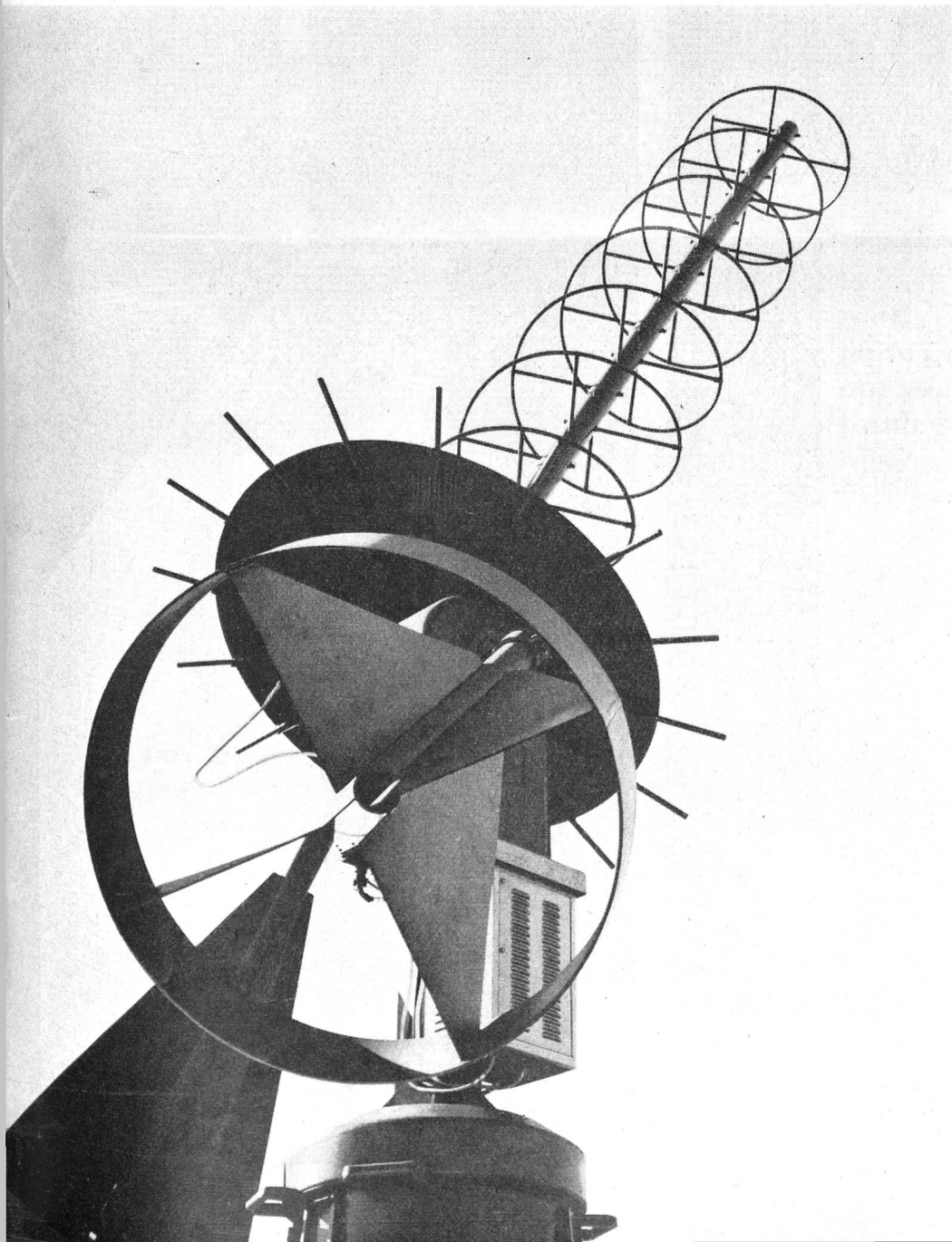
Wendelantenne für den Empfang von Bildern der Wettersatelliten der NASA
