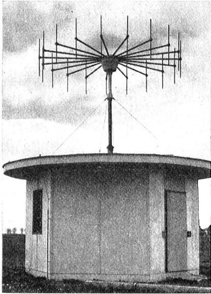
VHF - Peilanlage (Dopplerprinzip)
