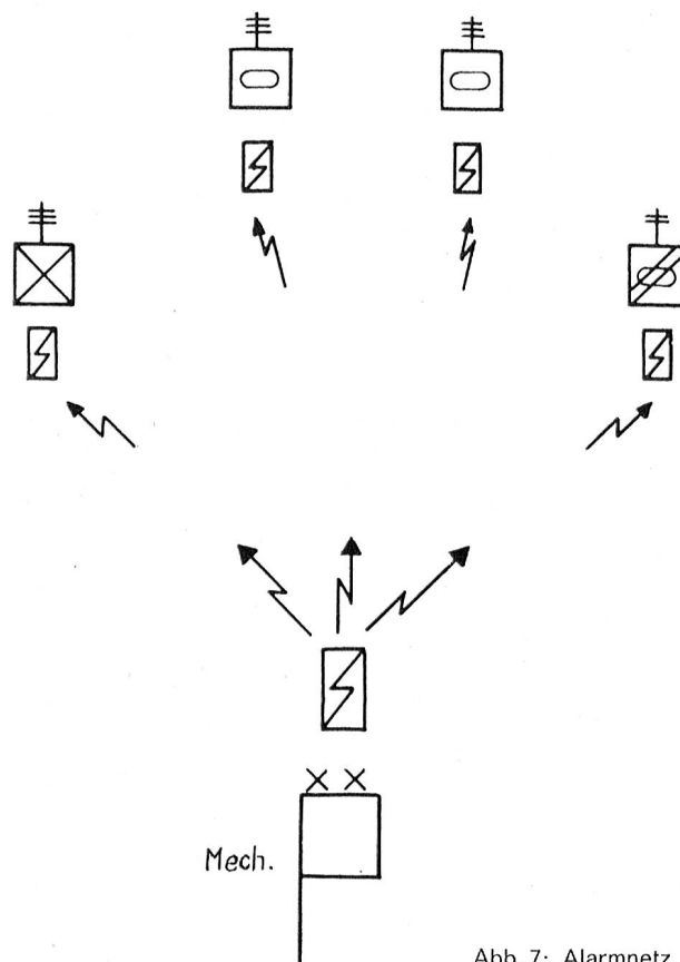
Abb. 7: Alarmnetz
