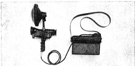
ALBIS-IR-Beobachtungsgerät «ARGUS»
