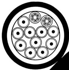
TYPE 1.2/4,4 MM \varnothing
