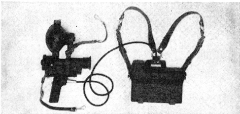
ALBIS-IR-Beobachtungsgerät «ARGUS»
