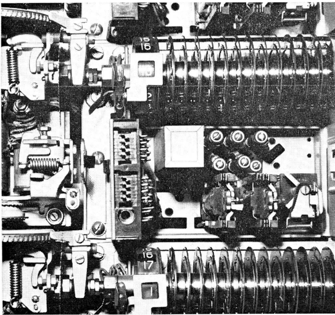
7-A Folgeschalter
