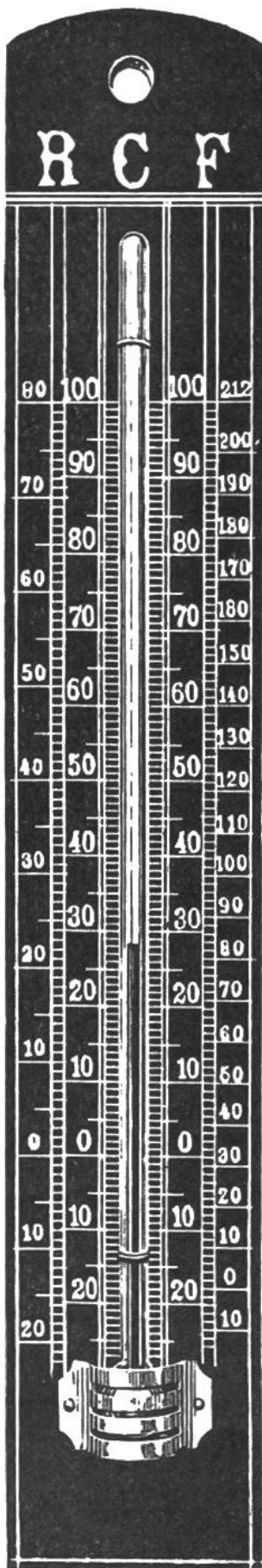
Réaumur-Celsius-Fahrenheit
