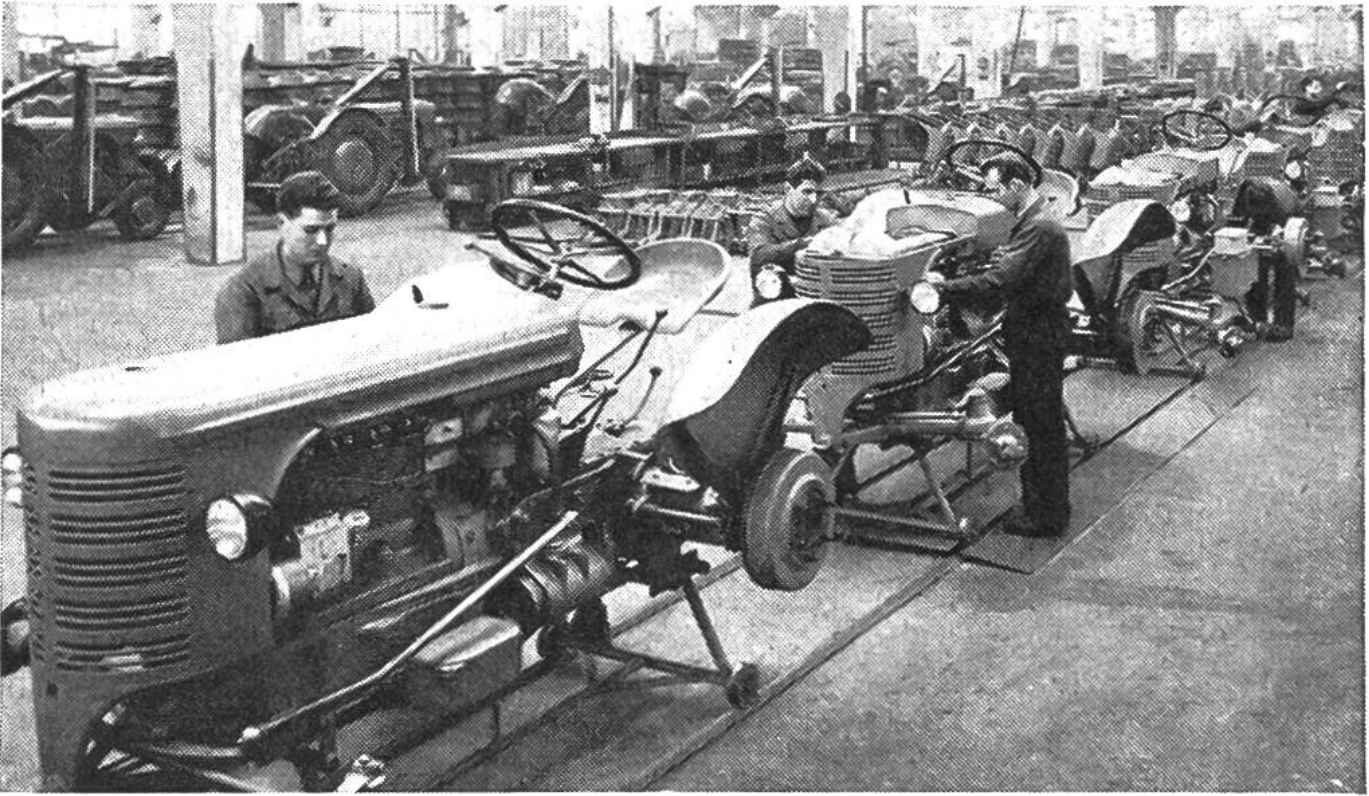
Blick in die Montagehalle einer schweizerischen Traktorenfabrik.
