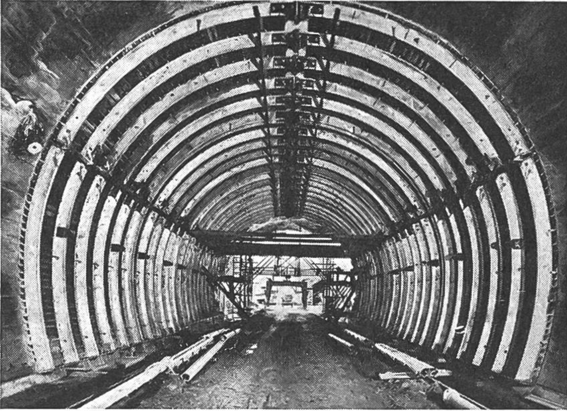
Stollenschalung aus Aluminiumlegierungen für den neuen Kerenzberg-Tunnel.
