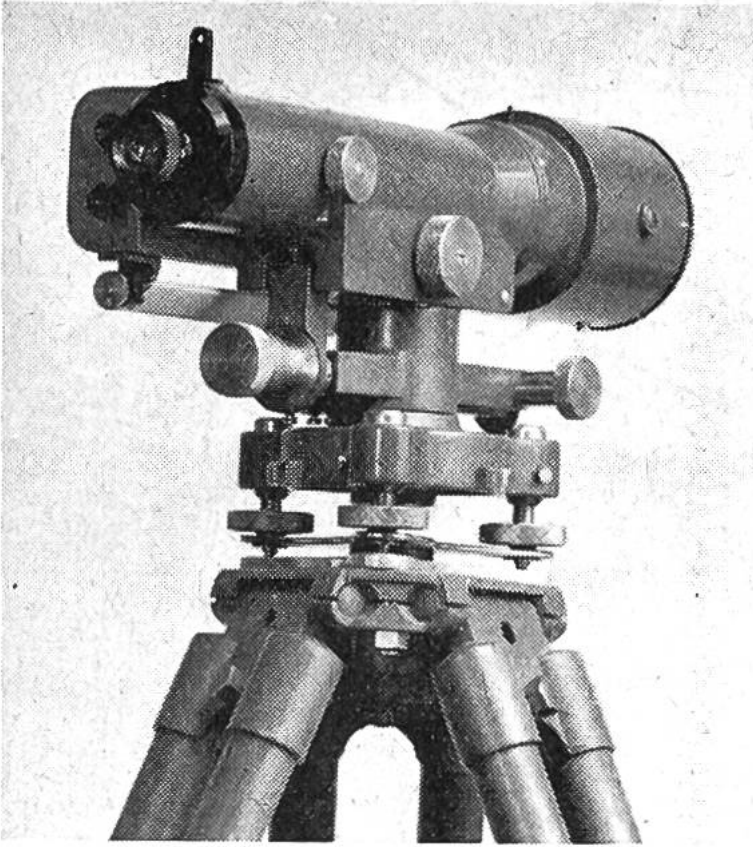
Nivellierinstrument.
